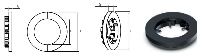
Bottom Cap
